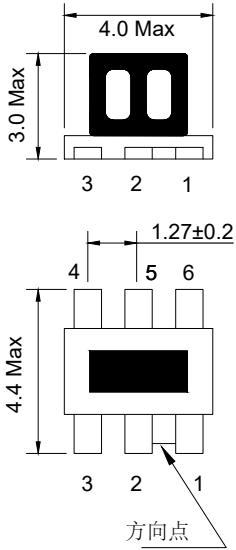
产品外形尺寸图(mm)
